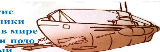
Торпедная атака
